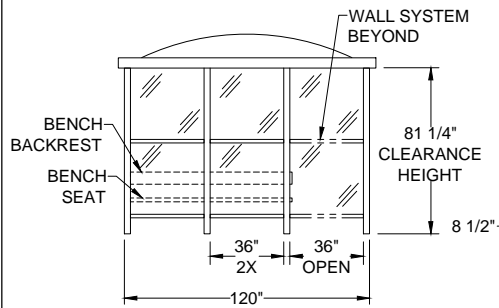
ELEVATION A
