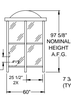
ELEVATION B
